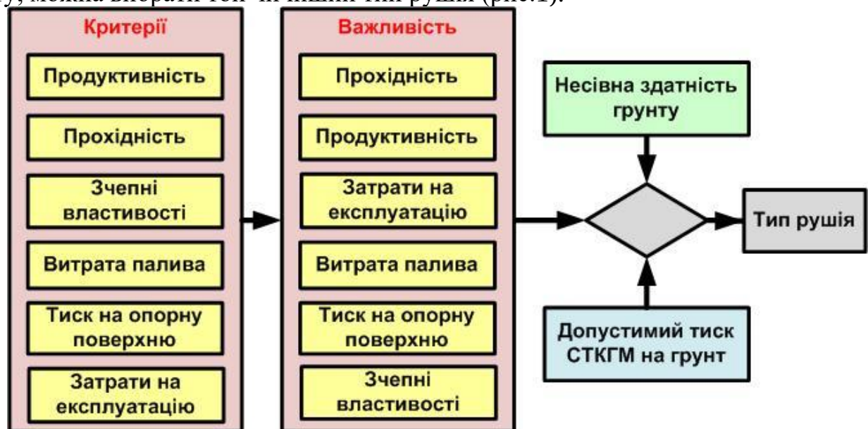
Рисунок. Алгоритм вибору типу рушія для СТКГМ
