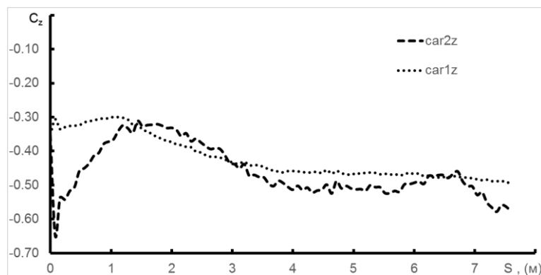
Рисунок 2.15 Коефіцієнт підйимальної сили транспортних засобів
