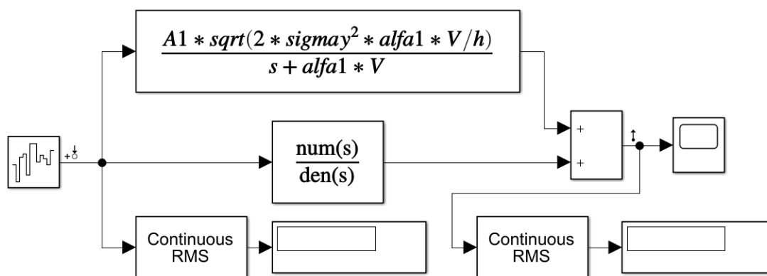
Рисунок 2 – Схема розрахунку конкретних значень мікропрофілю в програмному середовищі MATLAB Simulink
