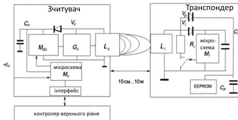
Рисунок 1 – Технологія RFID
