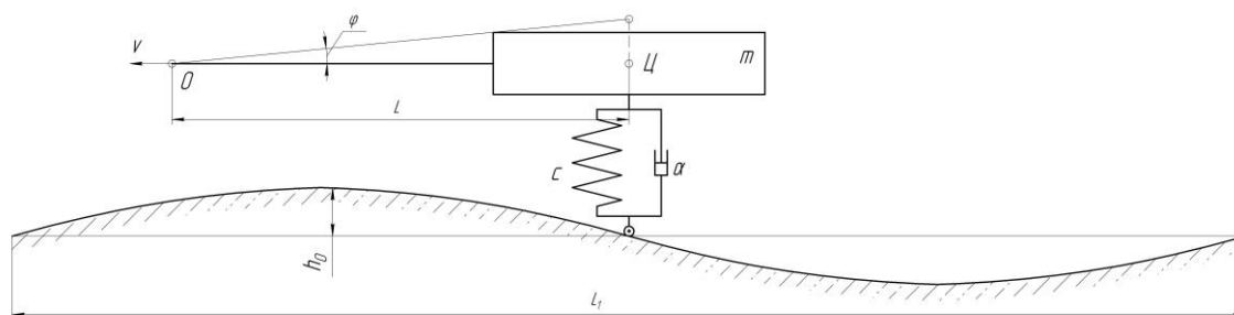
Рисунок 1 – Схема причепа
