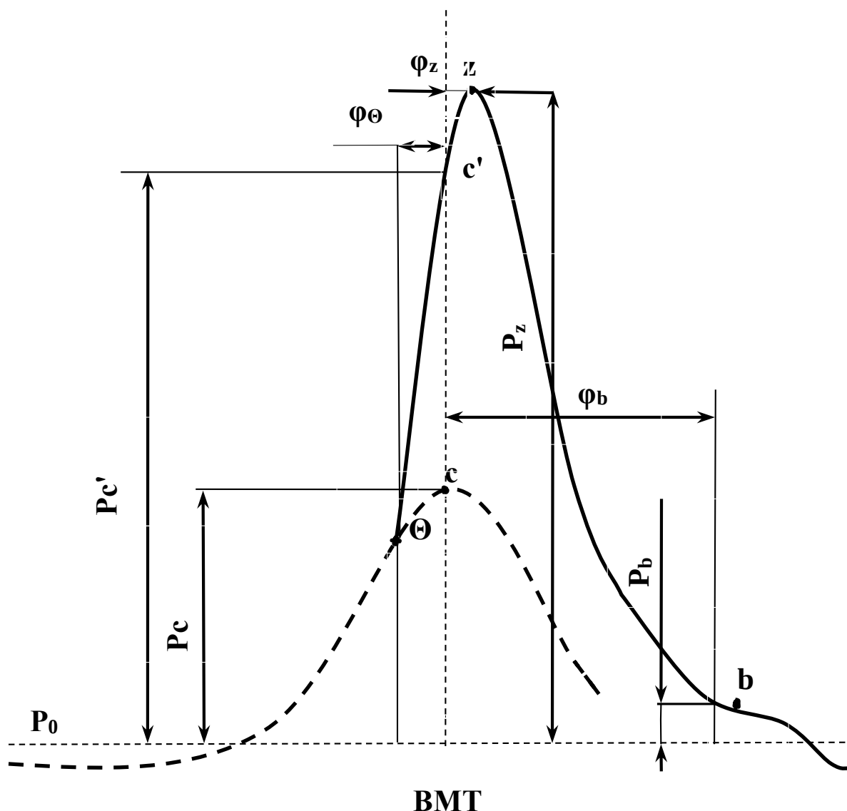
Рисунок 2 – Схема обробки індикаторної діаграми
