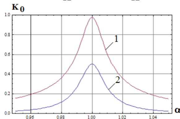
Рисунок 1. – Відносний коефіцієнт посилення реактивної потужності 1 – k_{12} = 1.0 и 2 – k_{12} = 0.16 .
