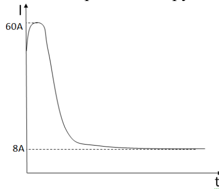
Рисунок 2 - Струм свічі накаливання
