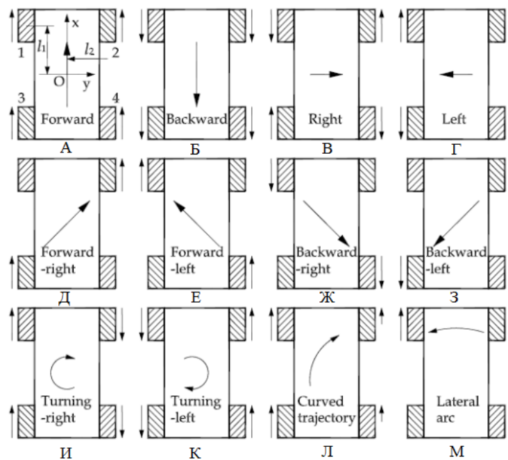
Рисунок 2 - Алгоритм руху платформи з колесами Mecanum
