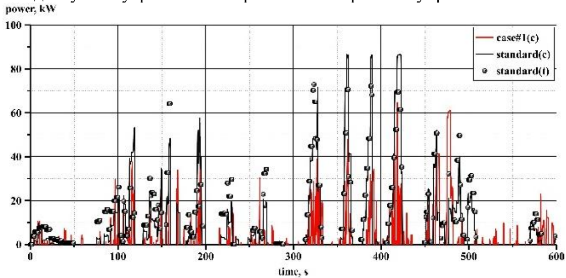
Рисунок 3 – Порівняння вимірювань потужності двигуна протягом діагностичного циклу, спричиненого виходом з ладу однієї з форсунок у модельованих та реальних умовах
