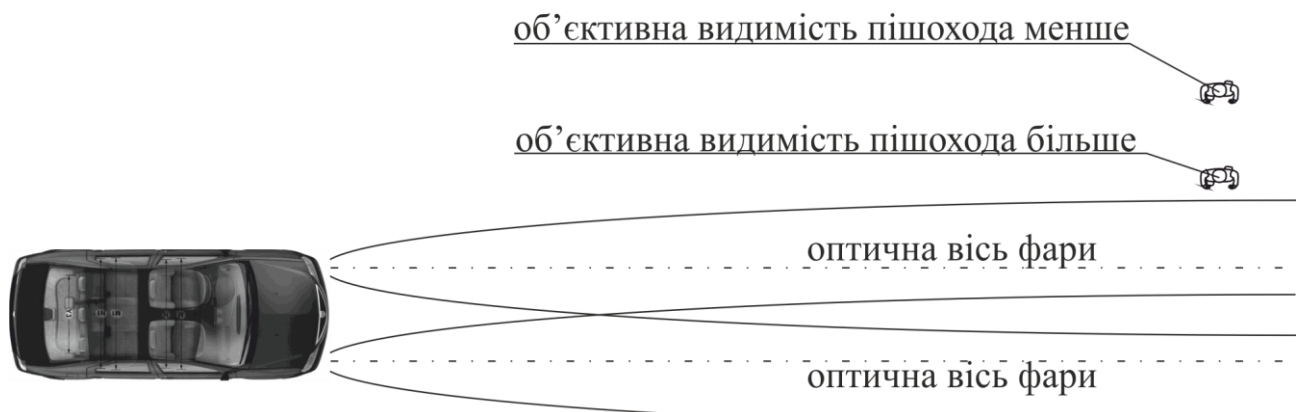
Рисунок 1. Зміна об'єктивної видимості пішохода в залежності від його розташування відносно оптичної осі фар автомобіля.
