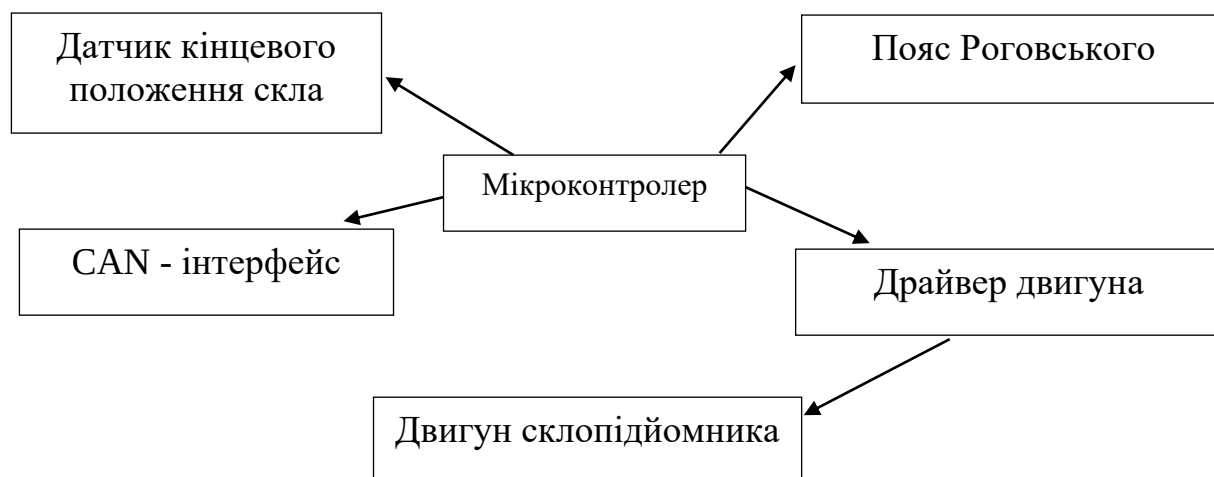
Рисунок 3 – Структурна схема системи керування електросклопідйомником
