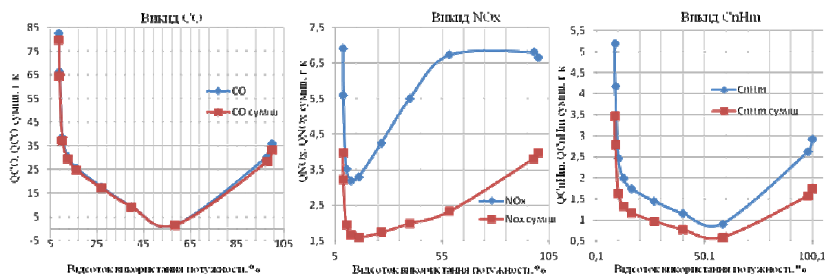
Рис. 2. Расчет количества вредных выбросов для Skoda Octavia
